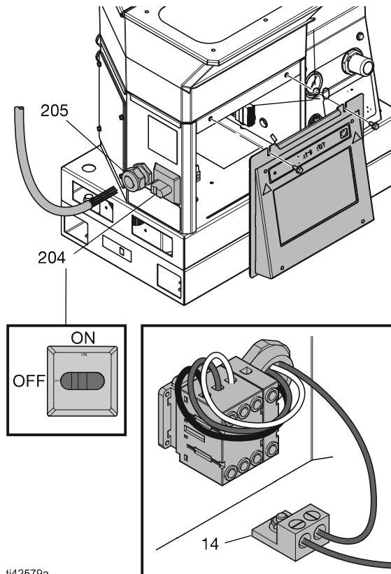
FIG. 8: Conexiones del cable eléctrico
