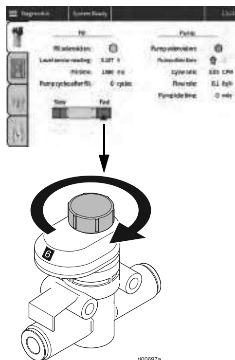
FIG. 67: Llenado rápido y restricción de aire
