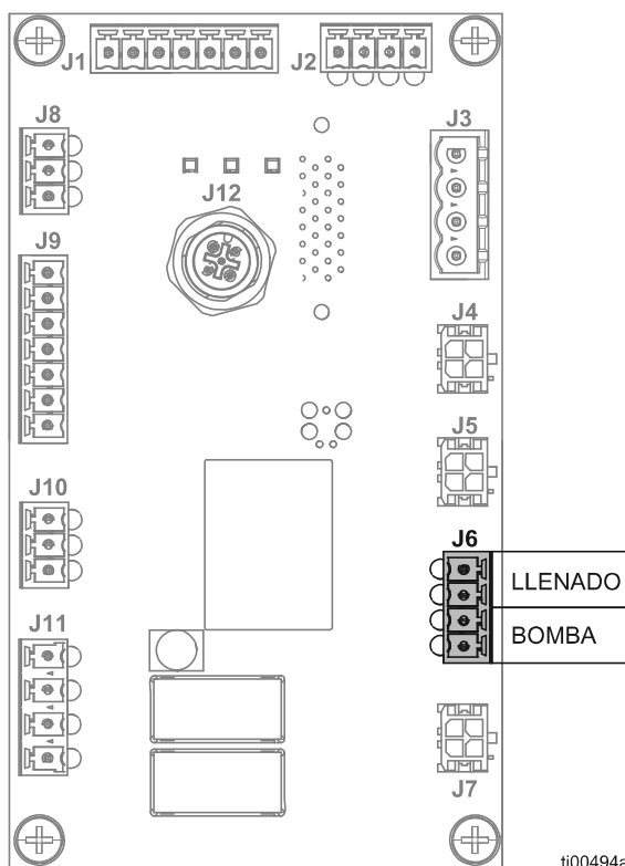
FIG. 76: Cableado del solenoide de control de aire (J6)
