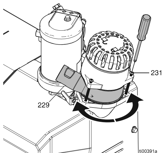
FIG. 2: Ajuste de la entrada del embudo
