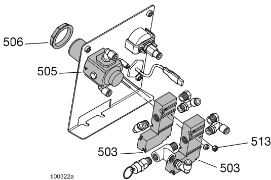
FIG. 74: Conjunto de control de aire
