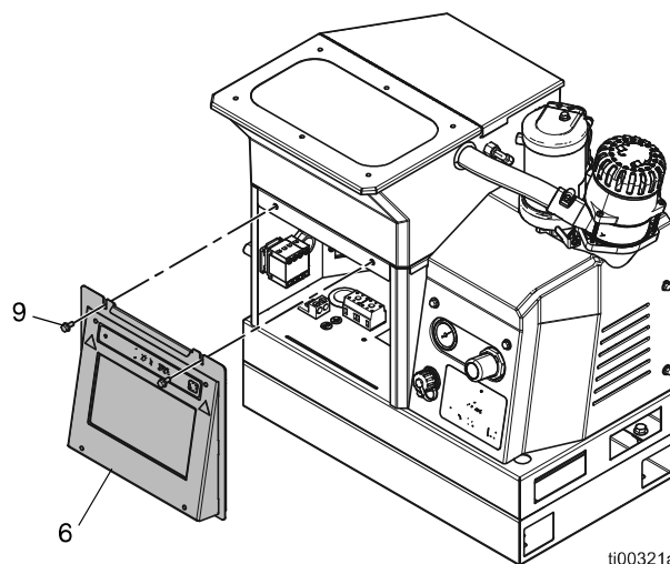
FIG. 69: Acceso al armario eléctrico
