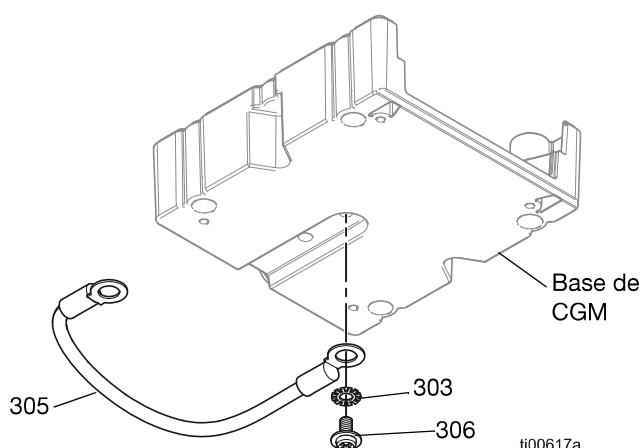
FIG. 110: Cable de conexión a tierra del CGM
