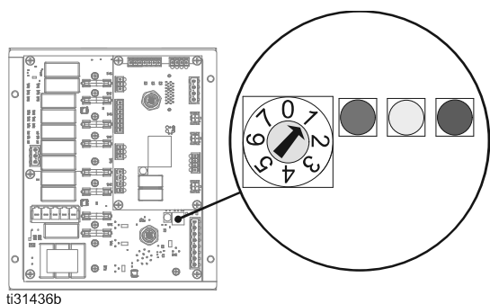
Fig. 92: Posición del dial de AMZ
