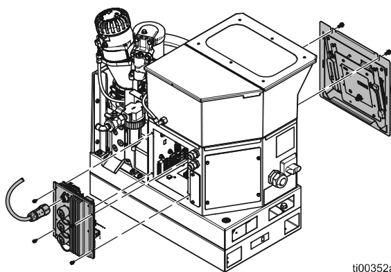
FIG. 91: Extracción de circuito impreso de AMZ
