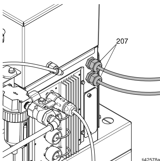
FIG. 12: Ubicación de prensacables de E/S
