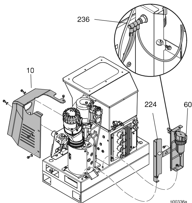
FIG. 68: Cubiertas para equipos
