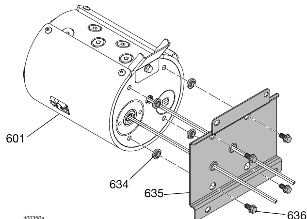
FIG. 78: Conjunto de placa del melter
