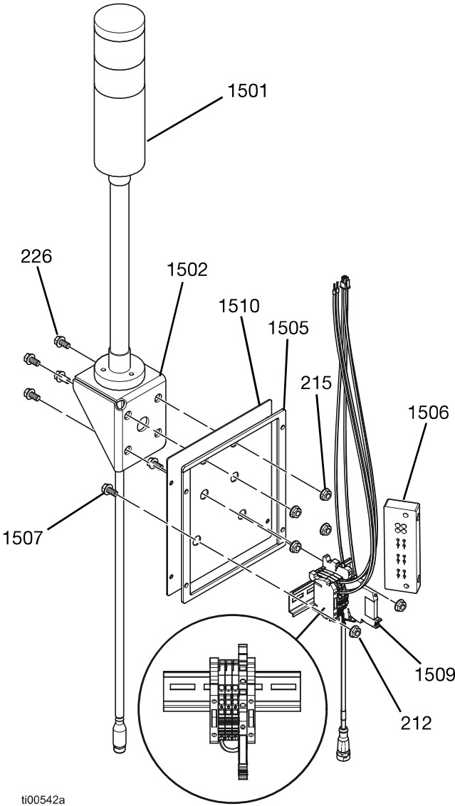
FIG. 104: Kit de torre de luces
