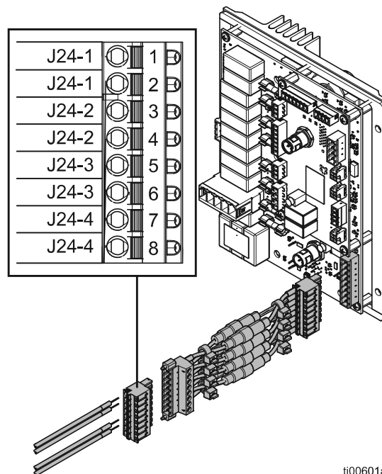
FIG. 89: Cableado de varilla de calentador (J24)
