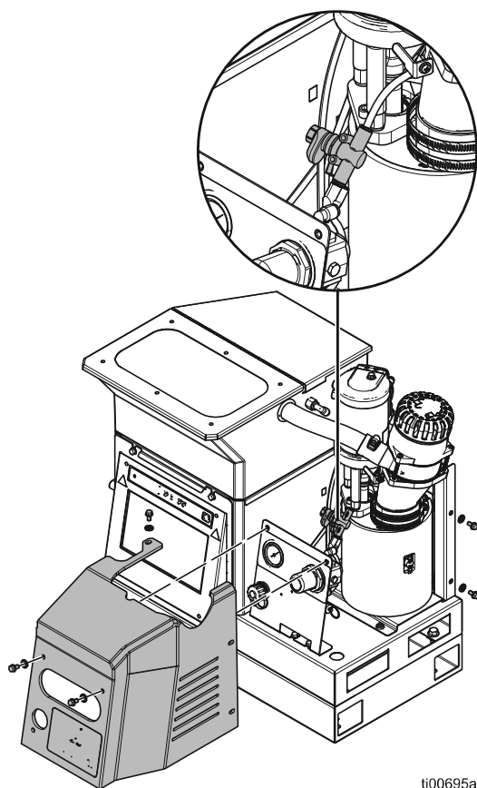
FIG. 65: Ubicación del venturi de aire
