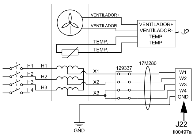
FIG. 99: Conexiones de alimentación eléctrica de entrada de 480 V y del ventilador del transformador (J2 y J22)
