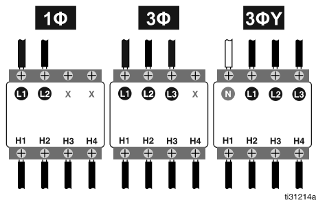
FIG. 7: Cableado de interruptor principal
