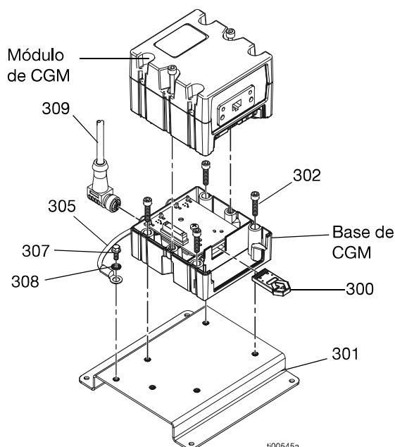
FIG. 111: Conjunto de CGM
