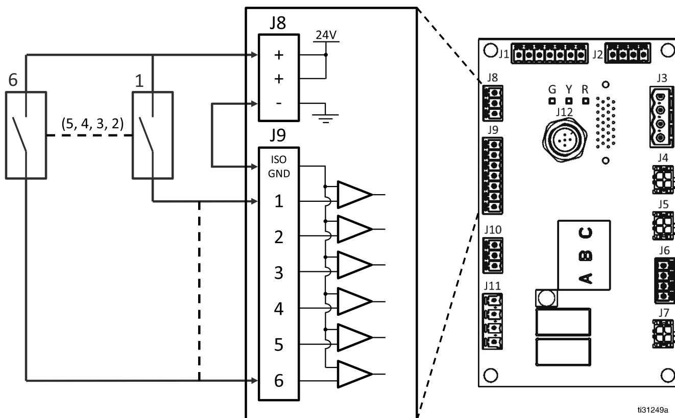
FIG. 14: Cableado (J8 y J9) de entradas de contacto seco (circuito abierto/cerrado)
