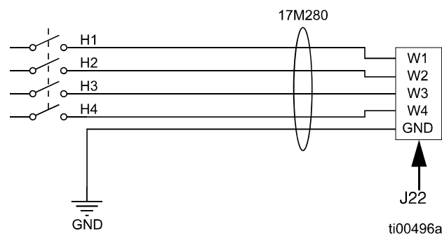
FIG. 98: Alimentación eléctrica de entrada de 240 V (J22)
