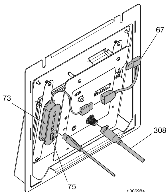
FIG. 118: Conexiones del ADM de 4 canales
