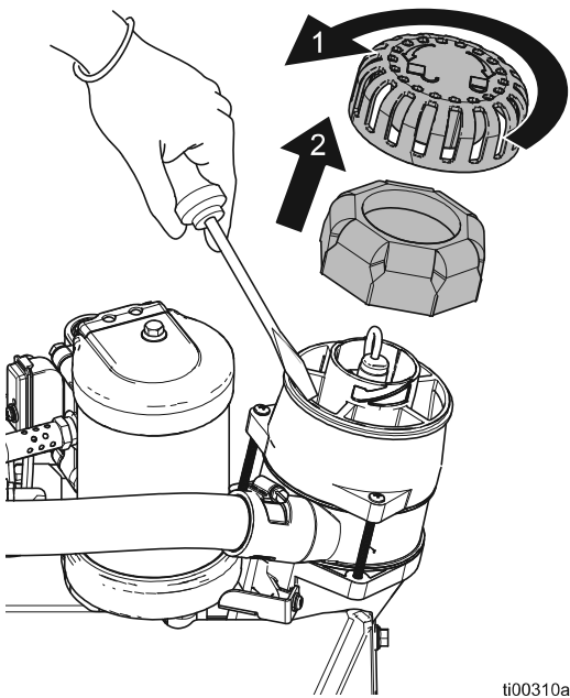
FIG. 29: Conjunto de tapa y filtro del embudo
