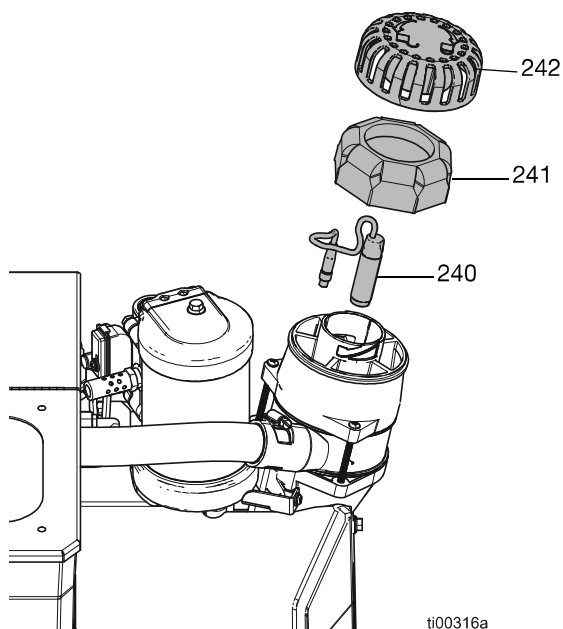
FIG. 70: Ubicación del sensor de nivel
