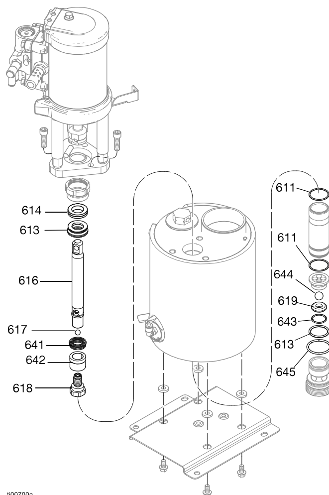
FIG. 102: Componentes de la bomba del melter
