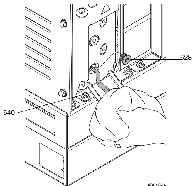
FIG. 1: Prueba de drenaje de aceite de la bomba del melter
