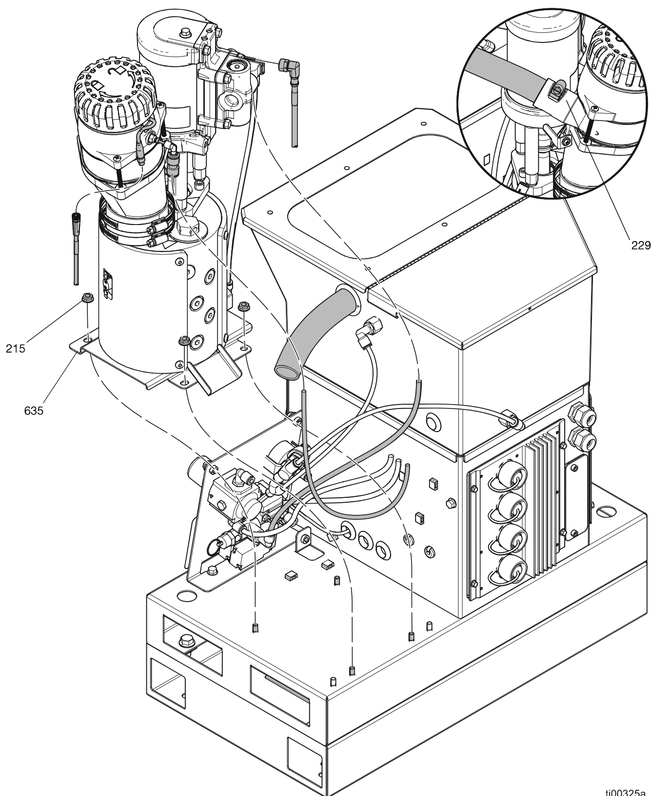
FIG. 77: Conexiones de la bomba del melter
