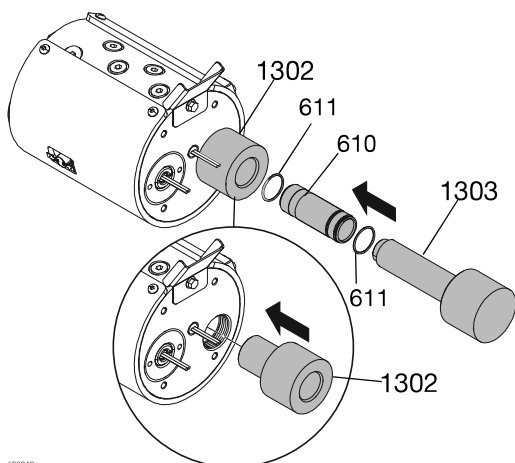
FIG. 84: Instalación del conjunto del cilindro
