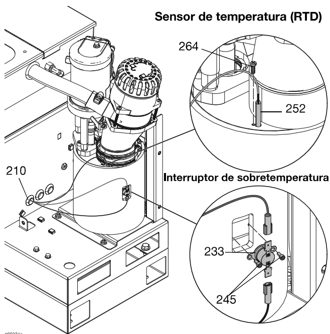
FIG. 72: Ubicación del sensor de temperatura y del interruptor de sobretensión
