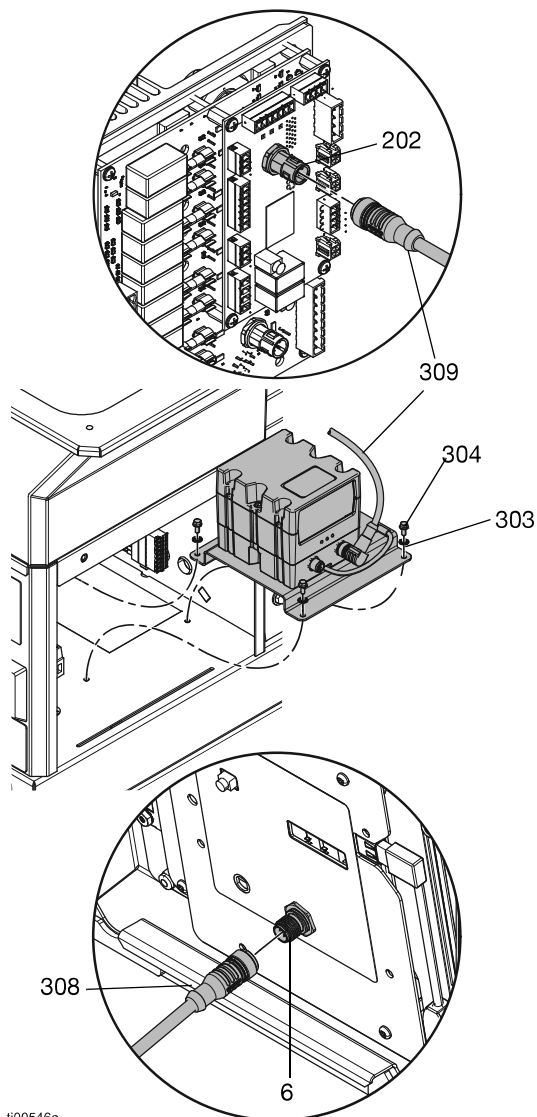
FIG. 112: Instalación y conexiones del CGM
