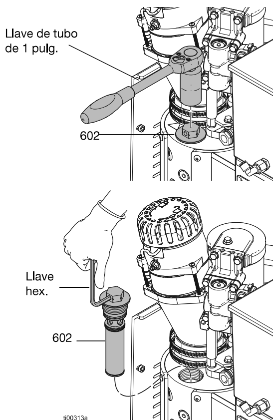
FIG. 31: Cambio del filtro de salida de la bomba
