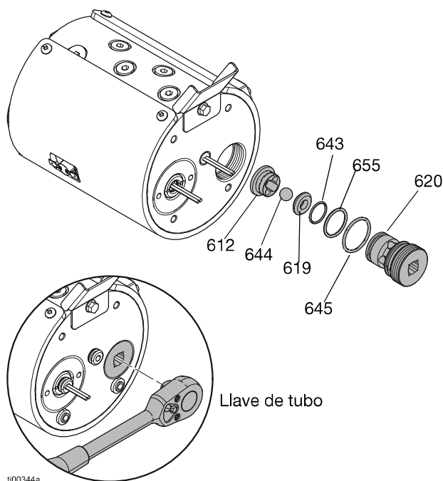
FIG. 82: Conjunto del alojamiento de entrada
