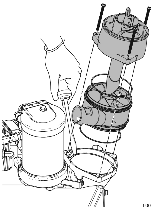
FIG. 30: Desmontaje del embudo
