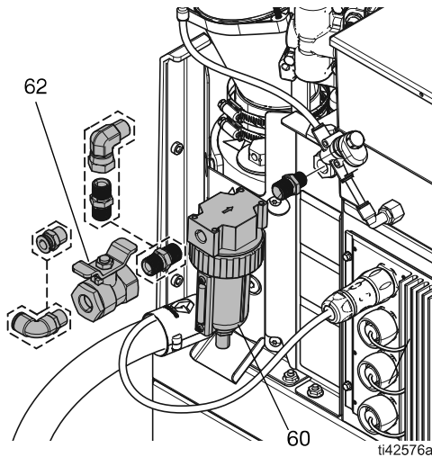
FIG. 5: Válvula de purga de aire e instalación del filtro de aire
