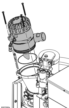
FIG. 22: Conjunto del embudo
