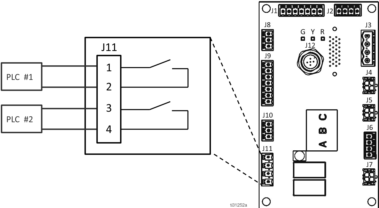
FIG. 15: Salidas de contactos secos (24 V CC/240 V CA, 2 A máx.) (J11)
