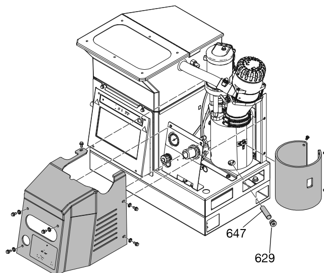
FIG. 32: Cambio del filtro de entrada de la bomba
