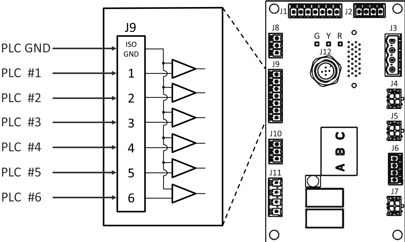
FIG. 13: Cableado de entradas digitales (J9)
