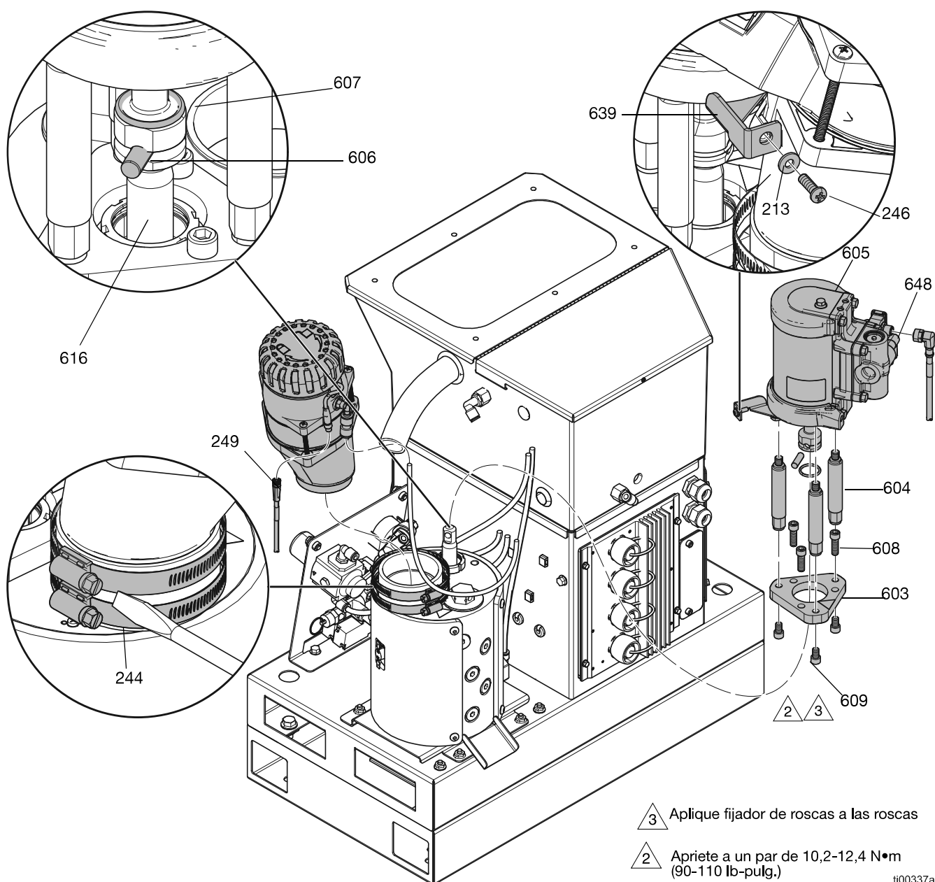
FIG. 79: Desmontaje del embudo y del motor neumático
