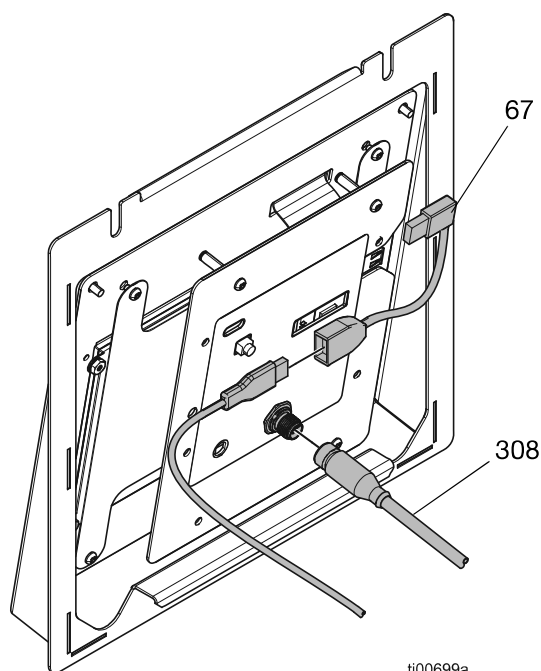
FIG. 117: Conexiones del ADM de 2 canales
