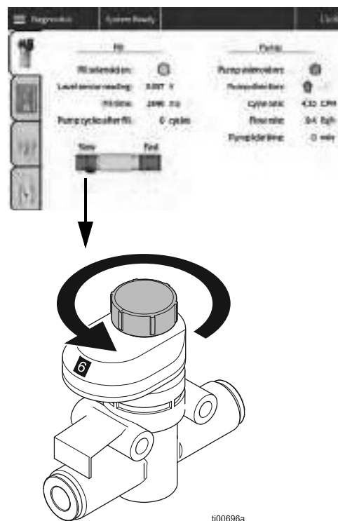
FIG. 66: Llenado lento y aumento de aire
