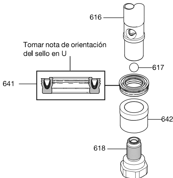
FIG. 81: Conjunto de pie del pistón
