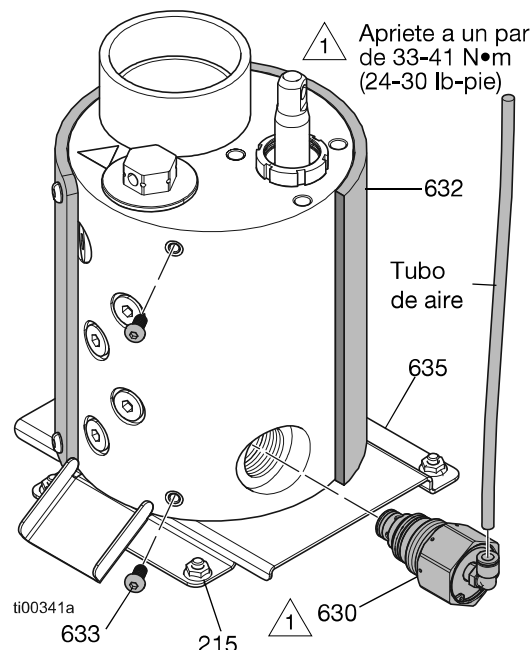
Fig. 87: Ubicación de la válvula de alivio de presión
