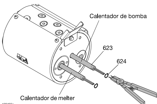
FIG. 88: Ubicación de varilla del calentador
