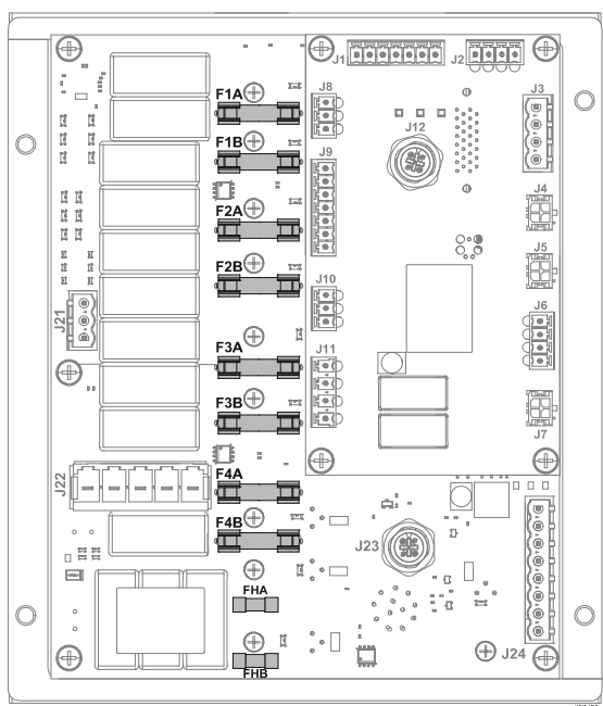
FIG. 90: Conexiones de fusibles de AMZ
