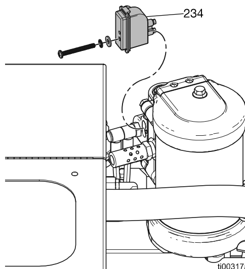
FIG. 71: Ubicación del interruptor de ciclo
