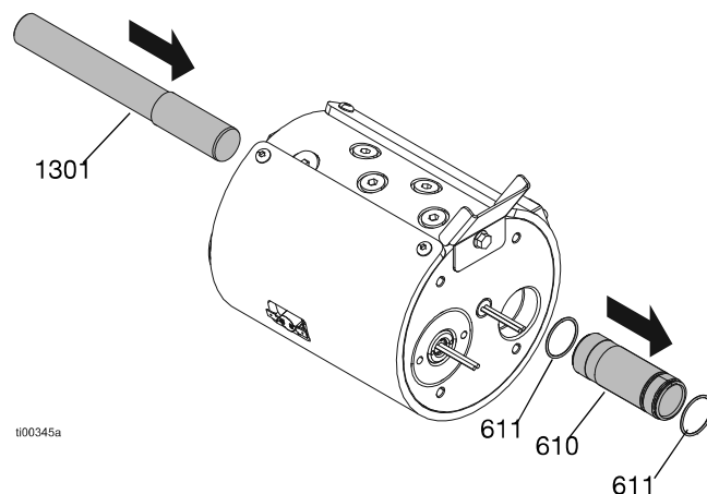
FIG. 83: Extracción del conjunto del cilindro
