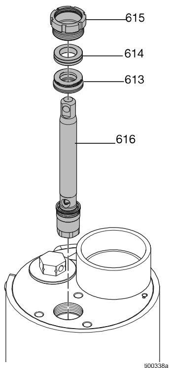
FIG. 80: Instalación del conjunto del eje del pistón
