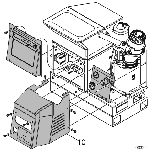
FIG. 75: Acceder a controles de aire
