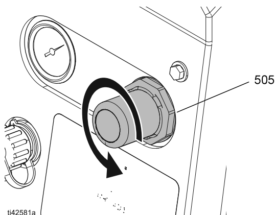
FIG. 18: Aumentar el ajuste del regulador de presión de aire
