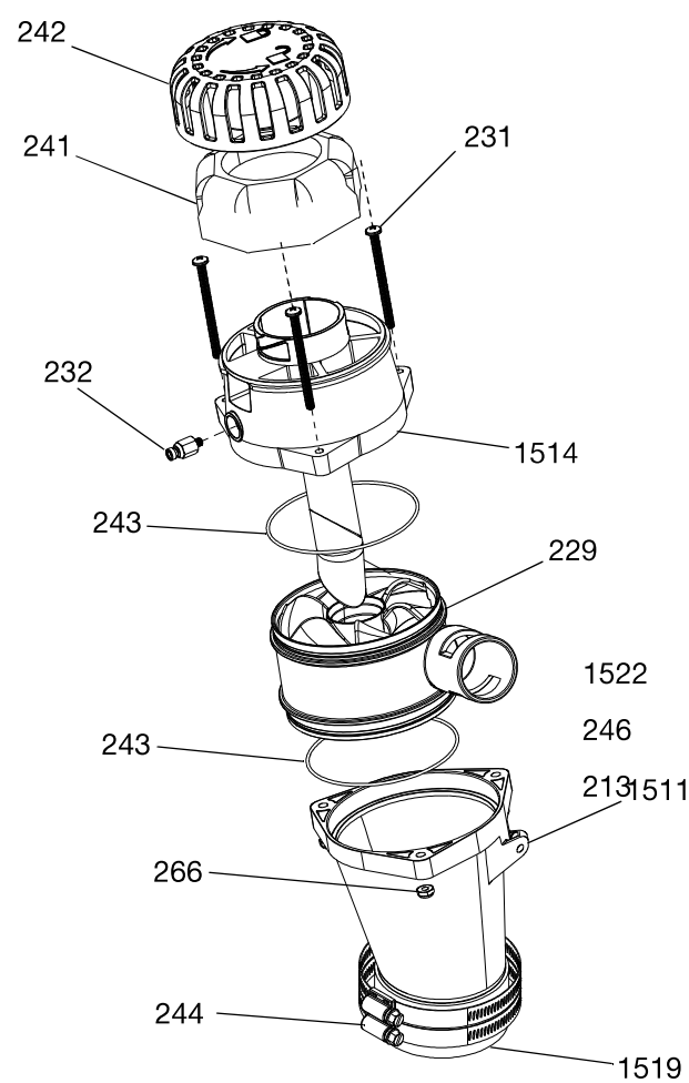
FIG. 103: Kit de conjunto de embudo
