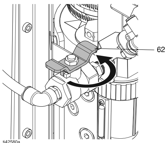
FIG. 17: Abrir la válvula de purga de aire
